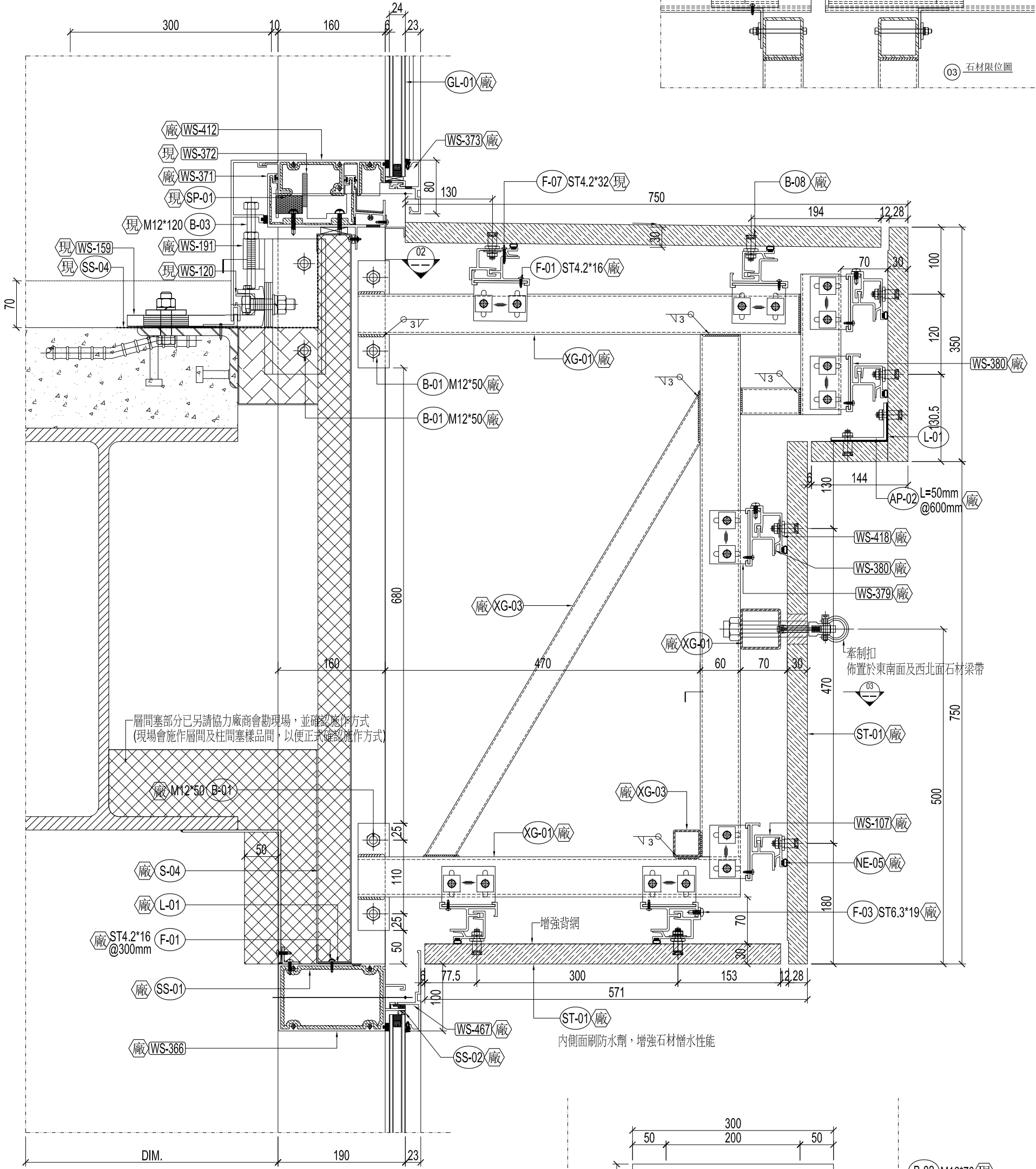
01 石材帷幕詳圖
