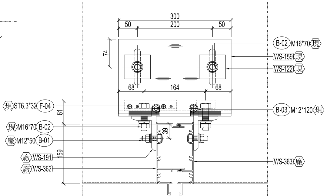
02 單元支座詳圖
