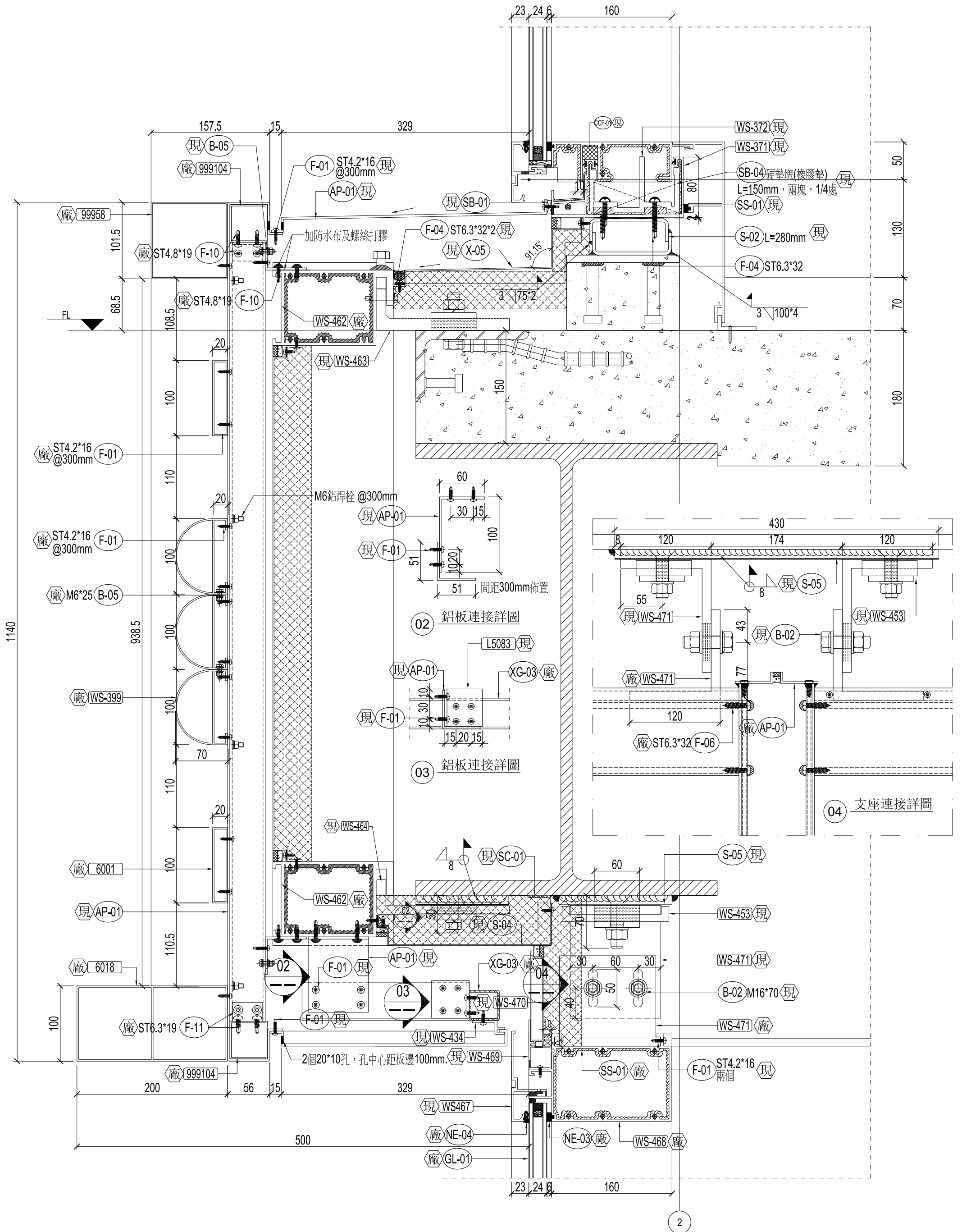
01 鋁板帷幕詳圖
