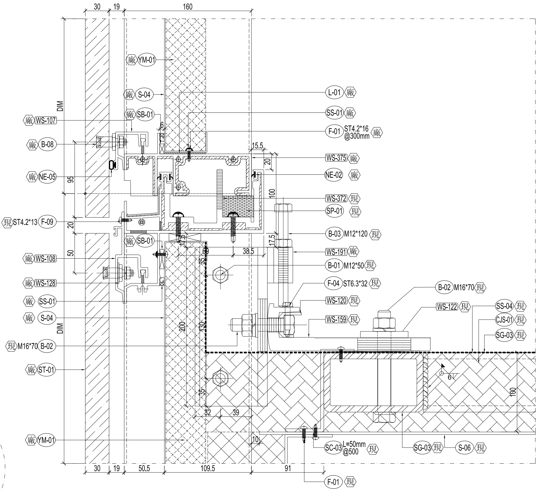
02 石材帷幕詳圖
