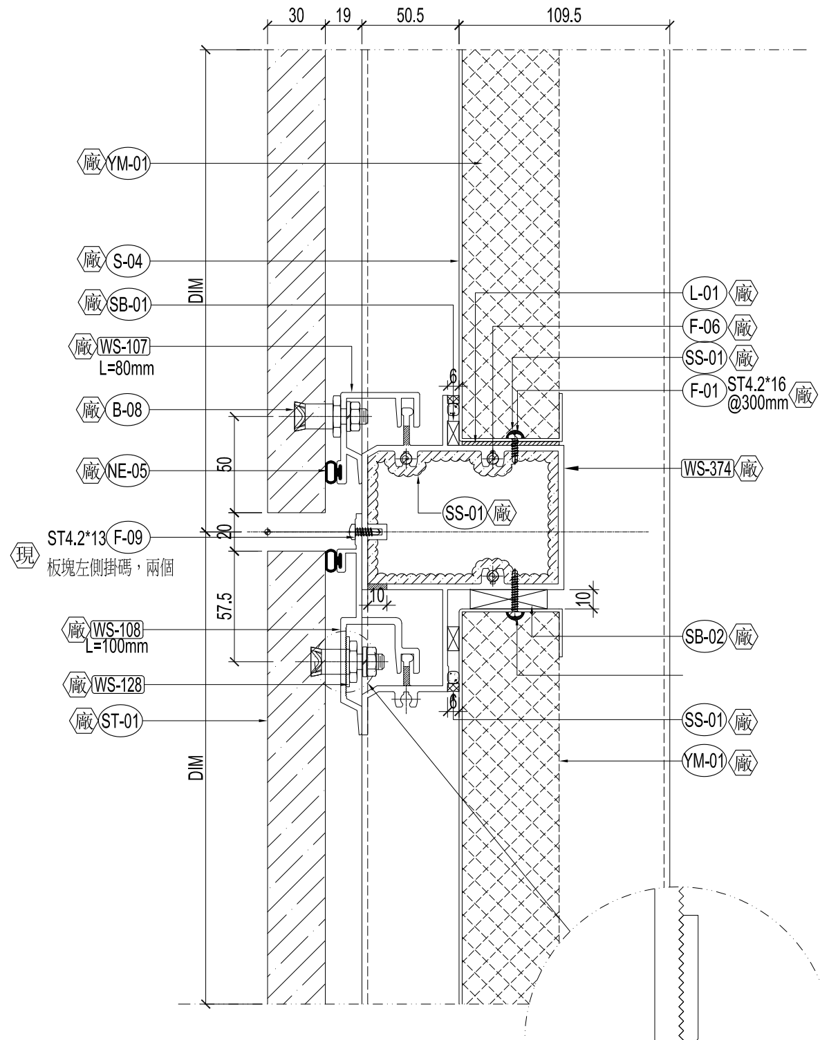
01 石材帷幕詳圖
