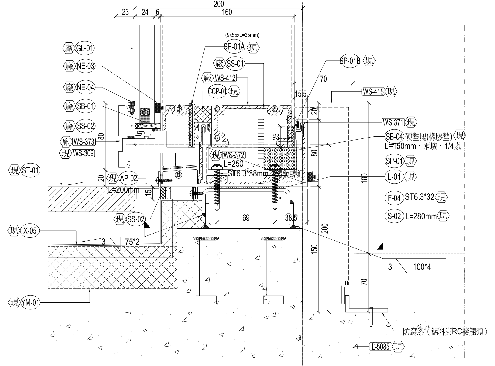
03 玻璃帷幕詳圖
