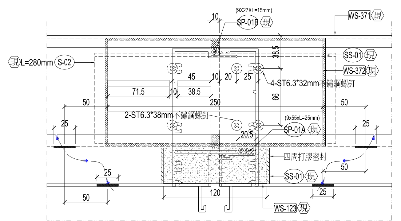
04 WS371支撐詳圖
