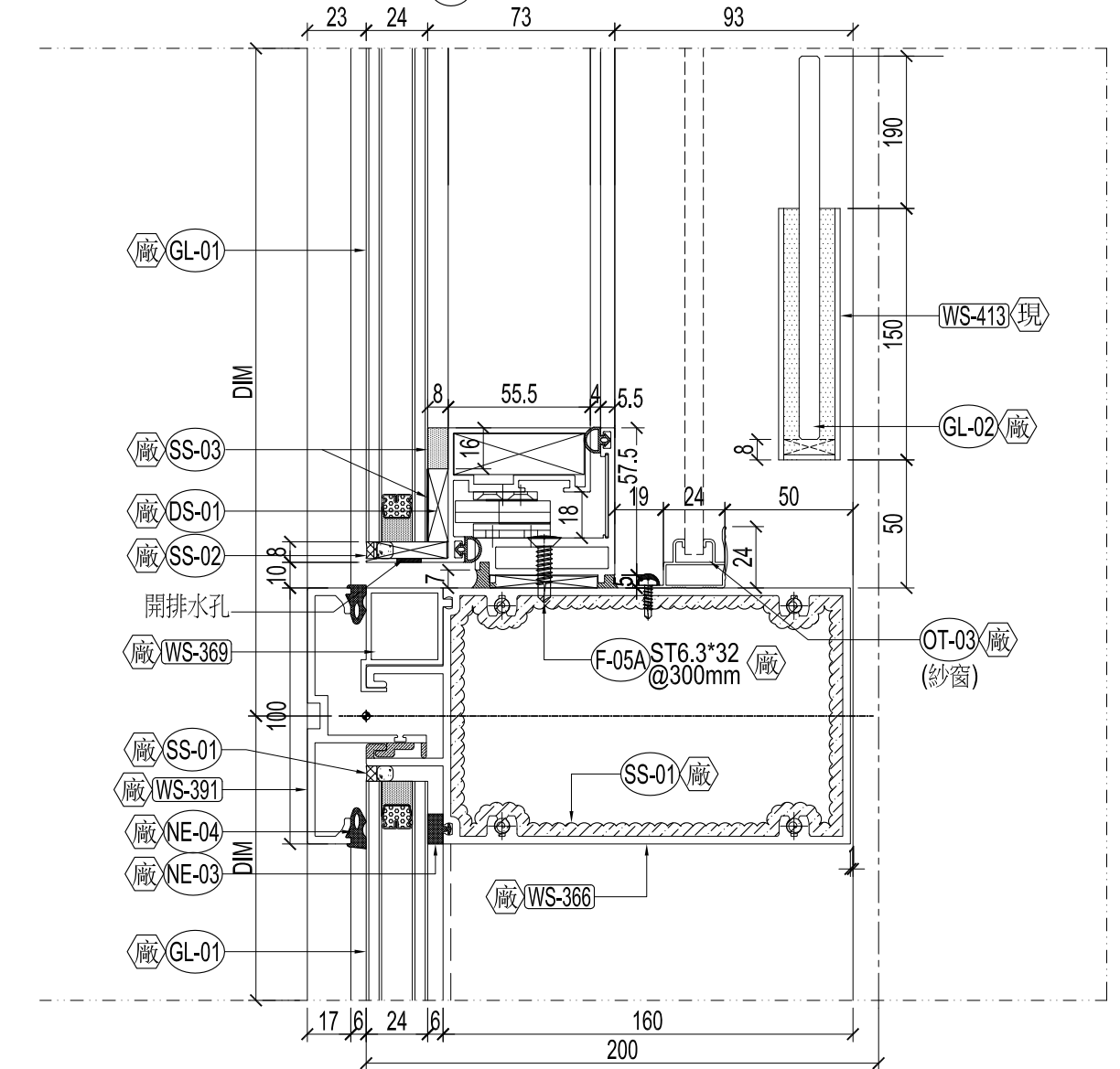
02 玻璃帷幕詳圖
