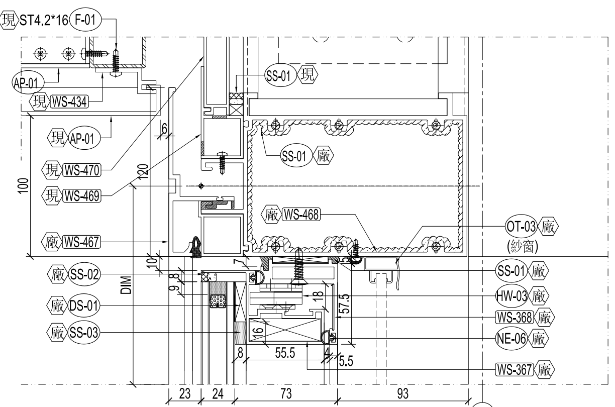
01 玻璃帷幕詳圖
