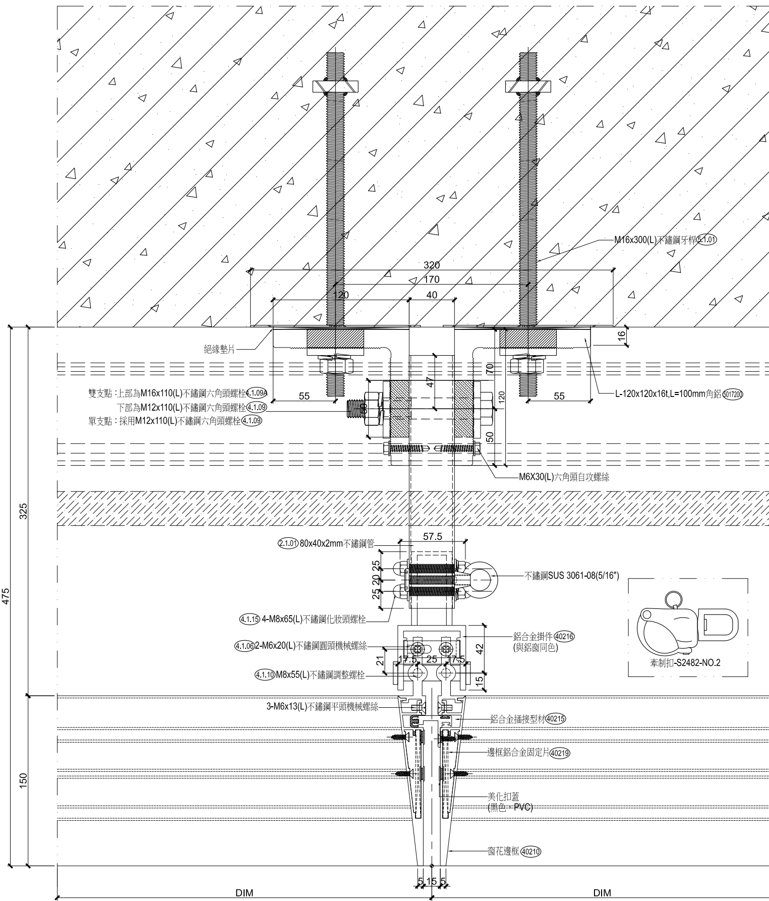
02 石材層間大樣 比例: 1:2
