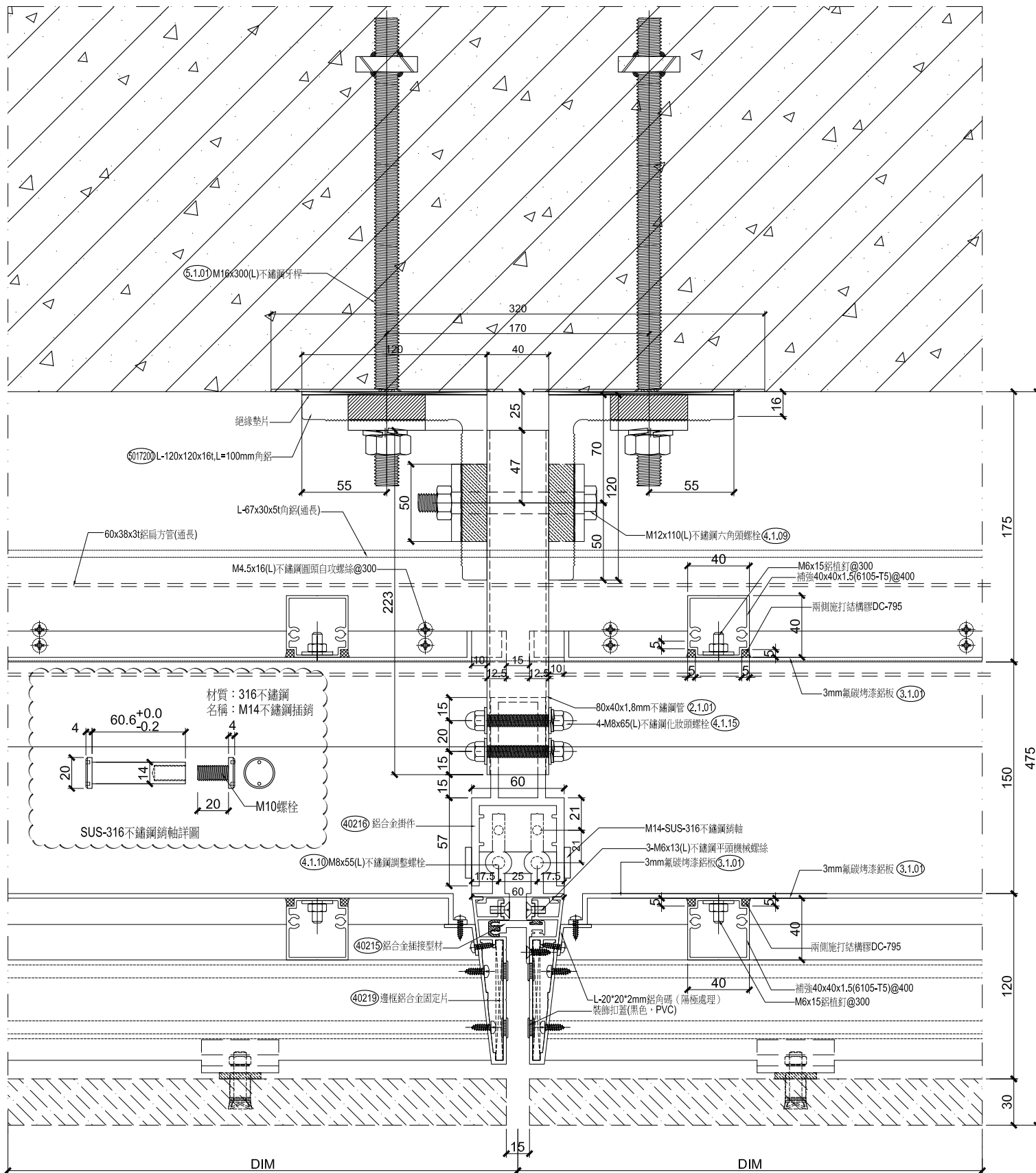
01 石材層間大樣 比例: 1:2
