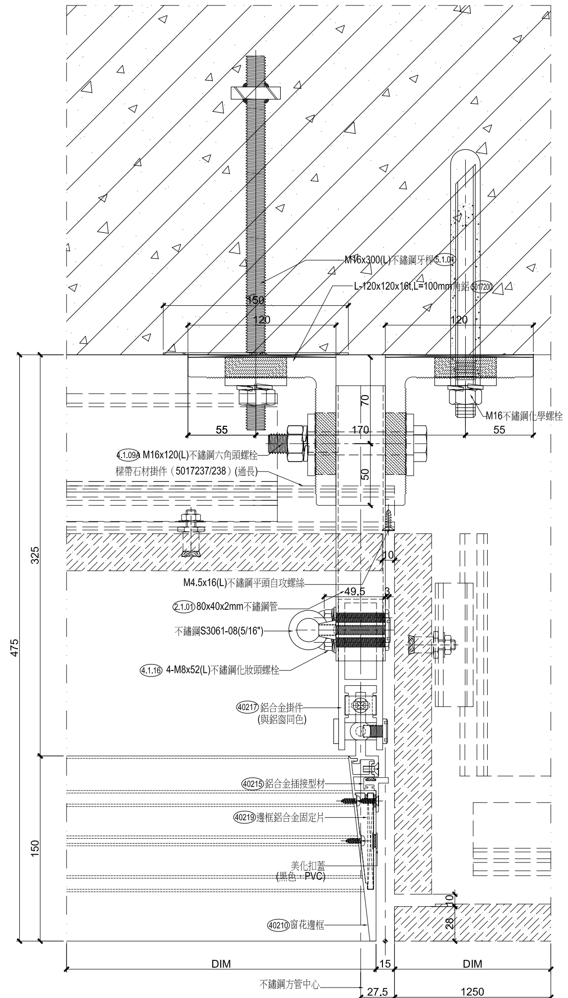
02 窗花層間大樣 比例： 1:2
