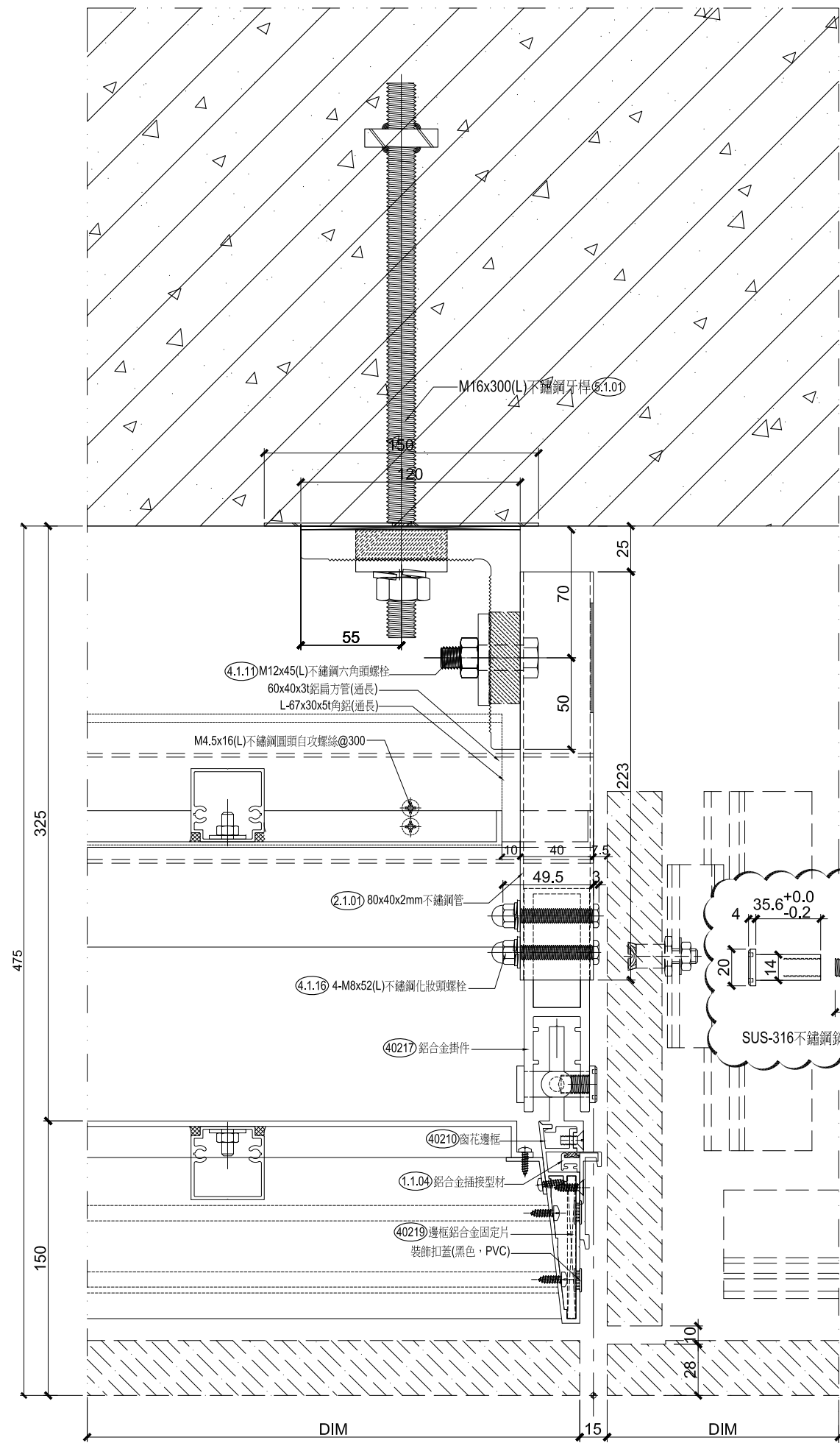
01 窗花層間大樣 比例： 1:2
