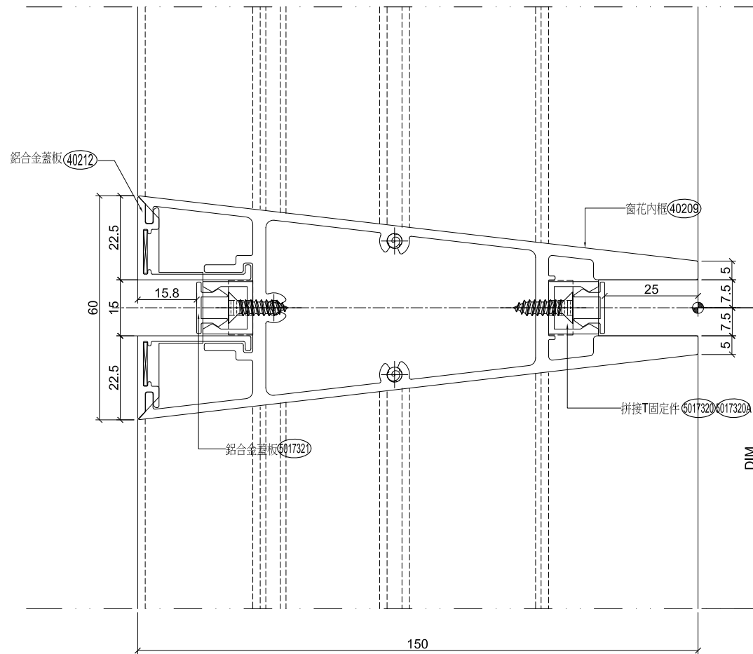
02 鋁合金窗花大樣 比例: 1:1
