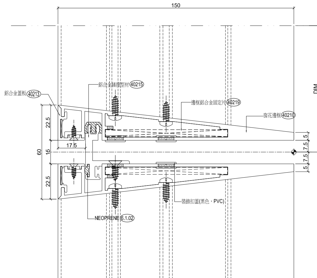
01 鋁合金窗花大樣 比例: 1:1
