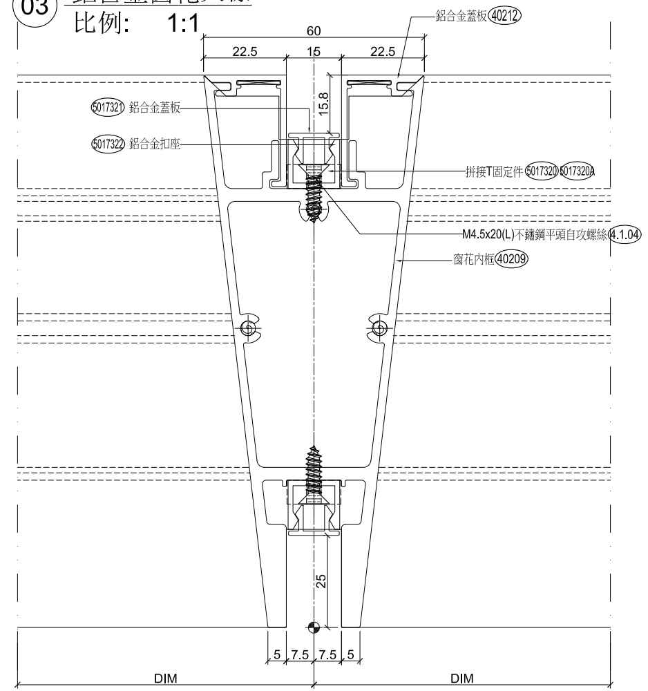
04 鋁合金窗花大樣 比例: 1:1
