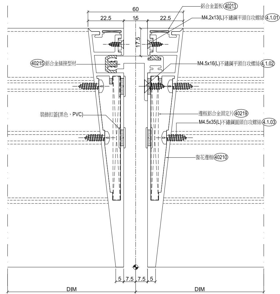
03 鋁合金窗花大樣 比例: 1:1
