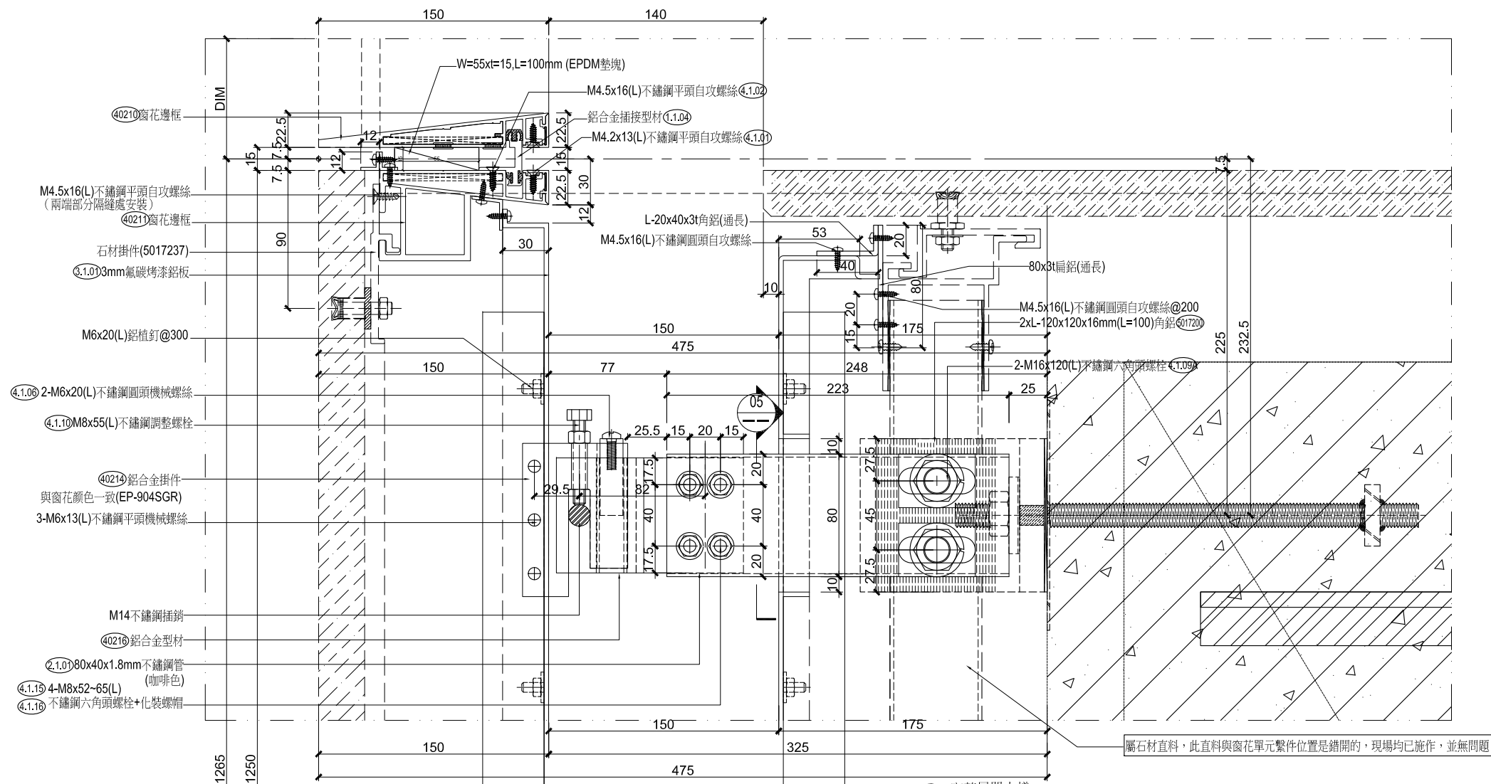
01 窗花層間大樣 比例: 1:2.5
