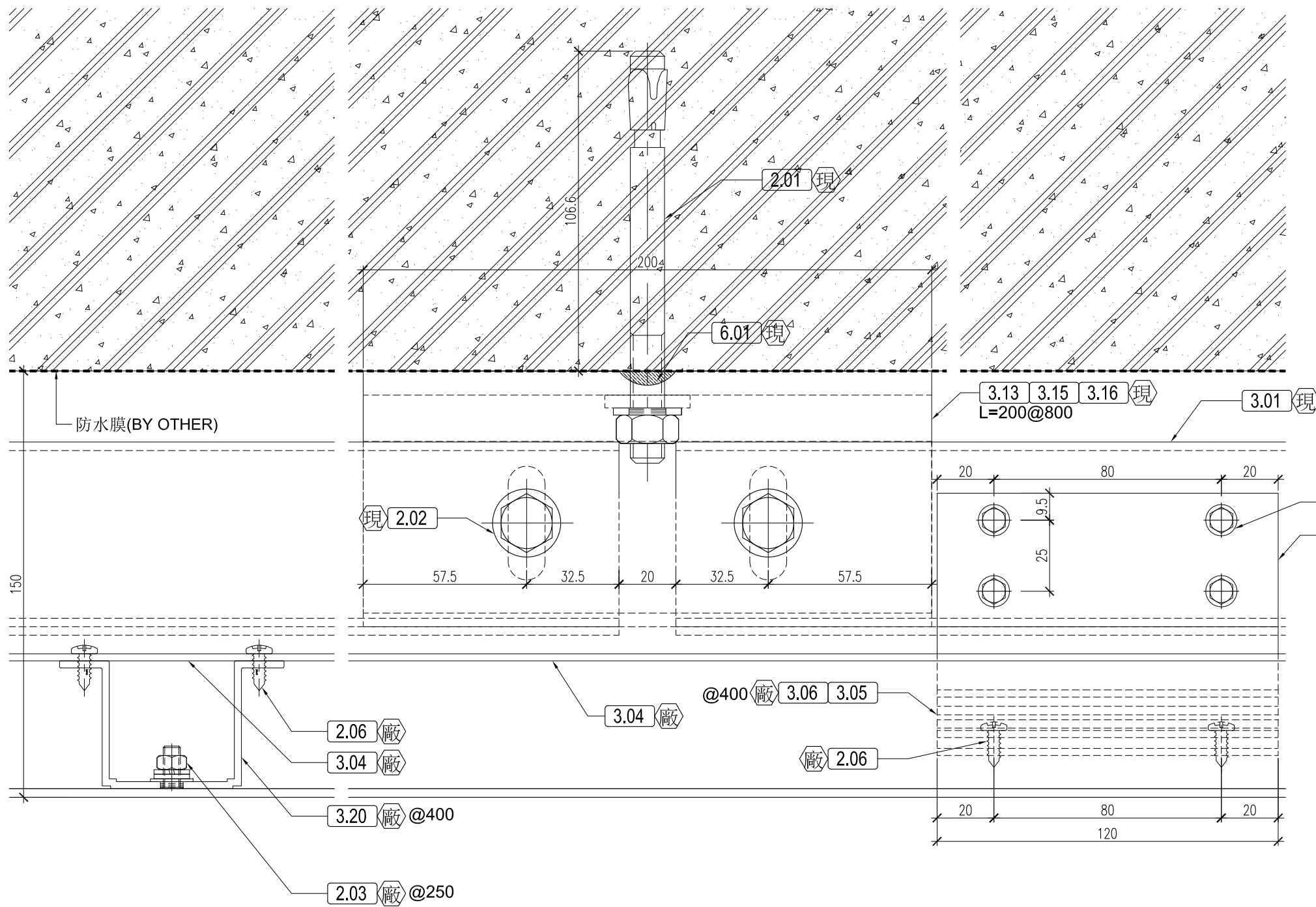
01 平剖細部詳圖 SCALE:1:2
