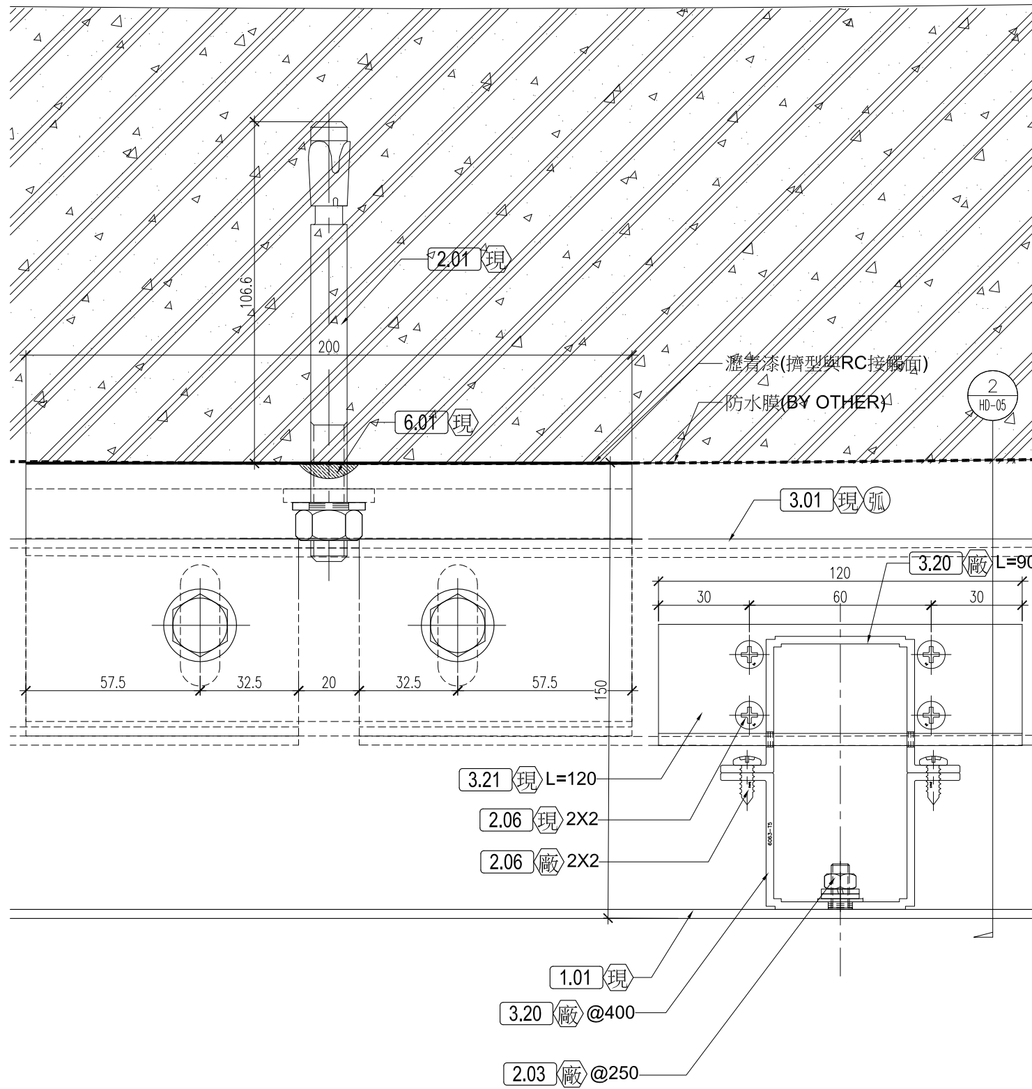
01 平剖細部詳圖 SCALE:1:2
