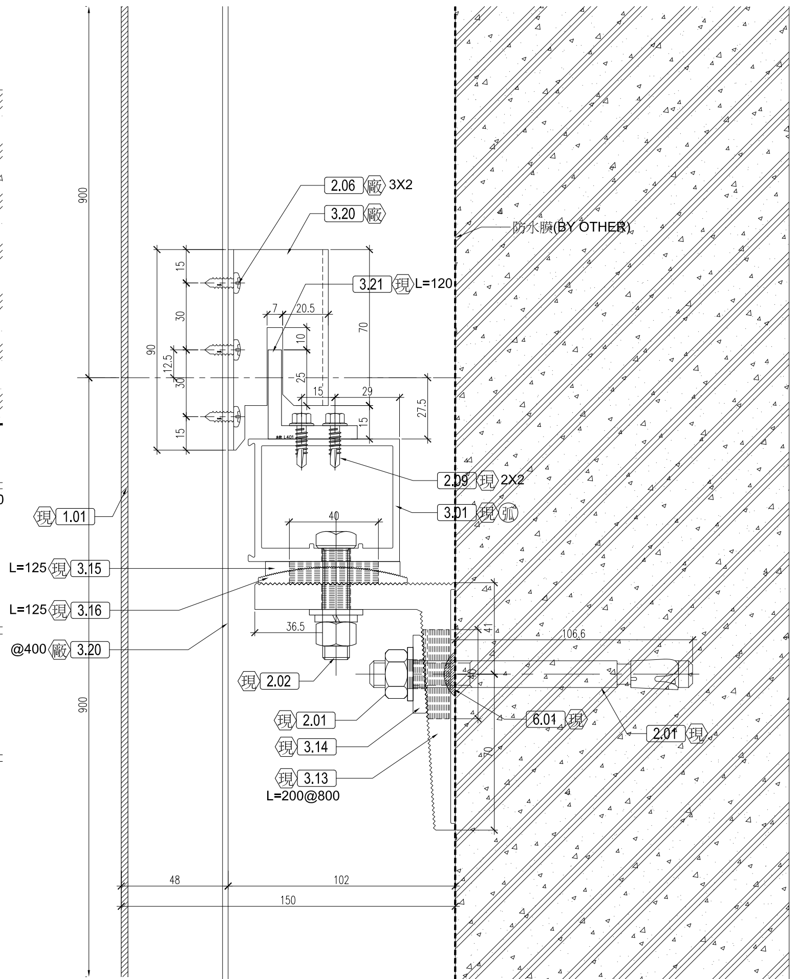
02 立剖細部詳圖 SCALE:1:2
