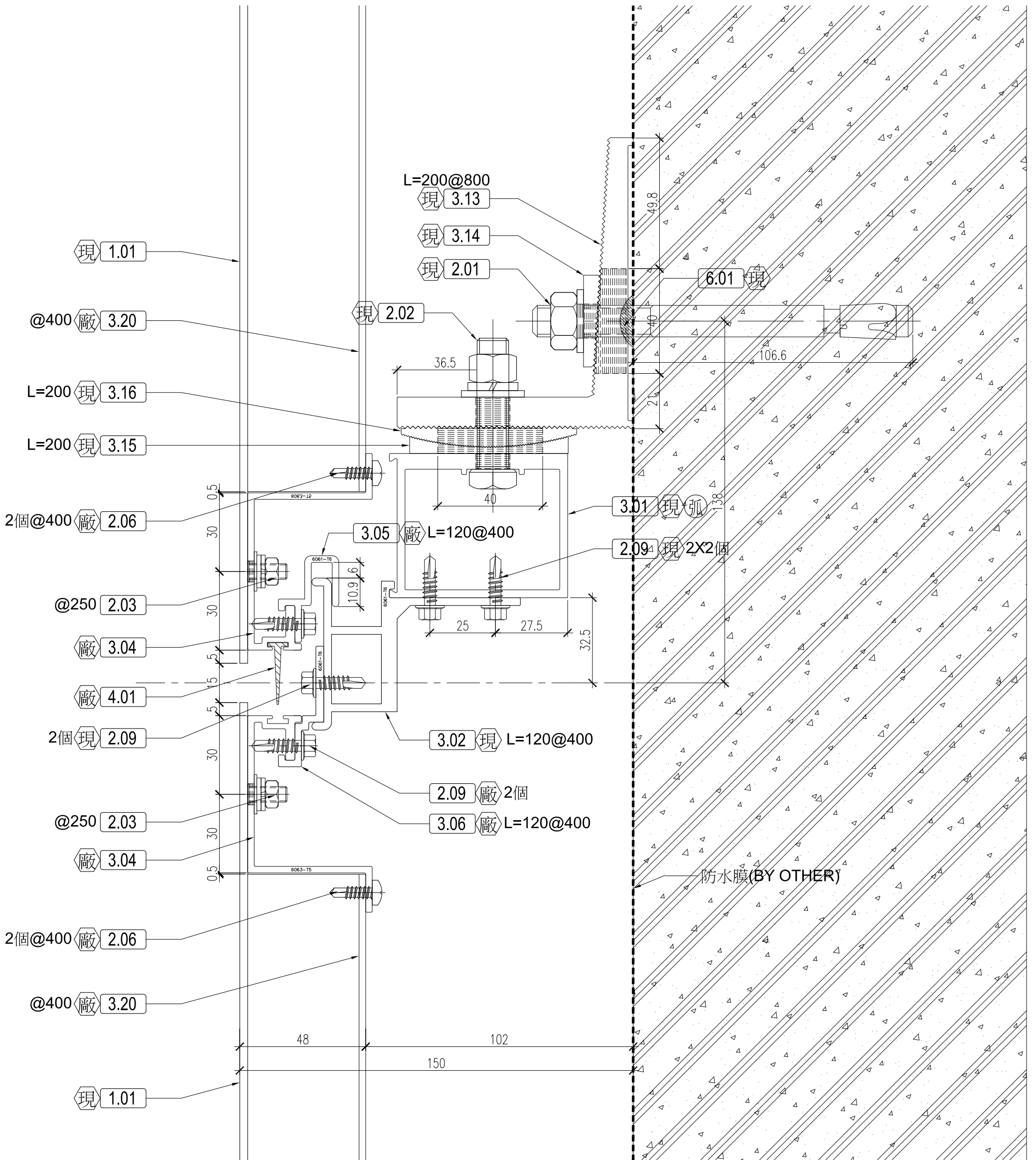
01 立剖細部詳圖 SCALE:1:2
