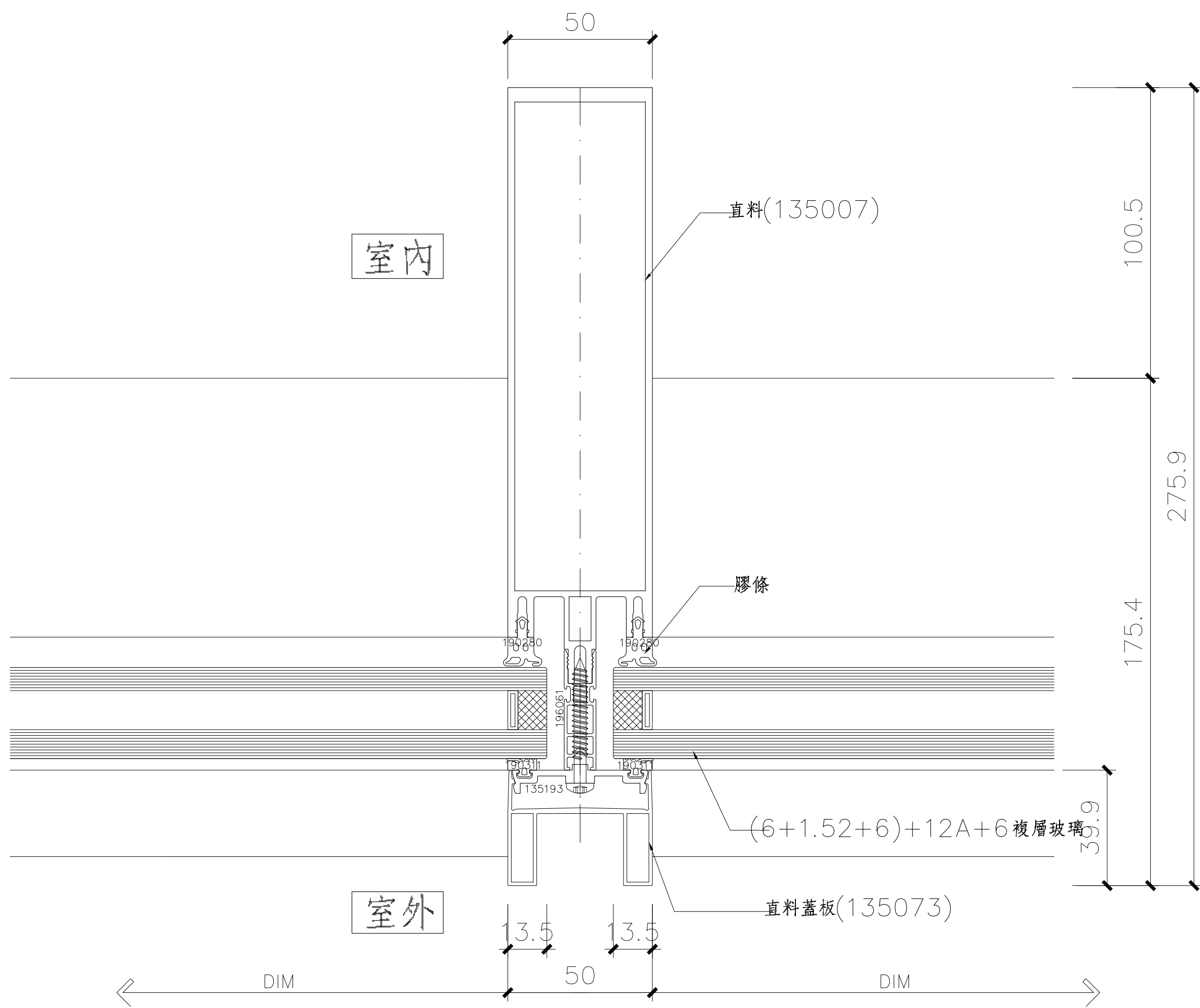
1 帷幕窗平斷面詳圖
