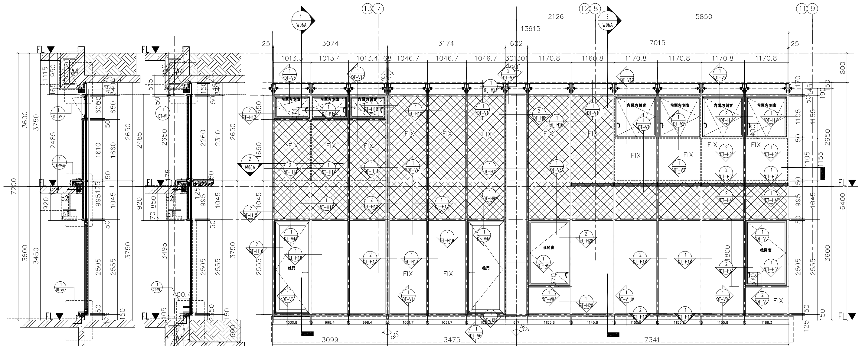
挑空區陽台帷幕窗外視展開立面圖
