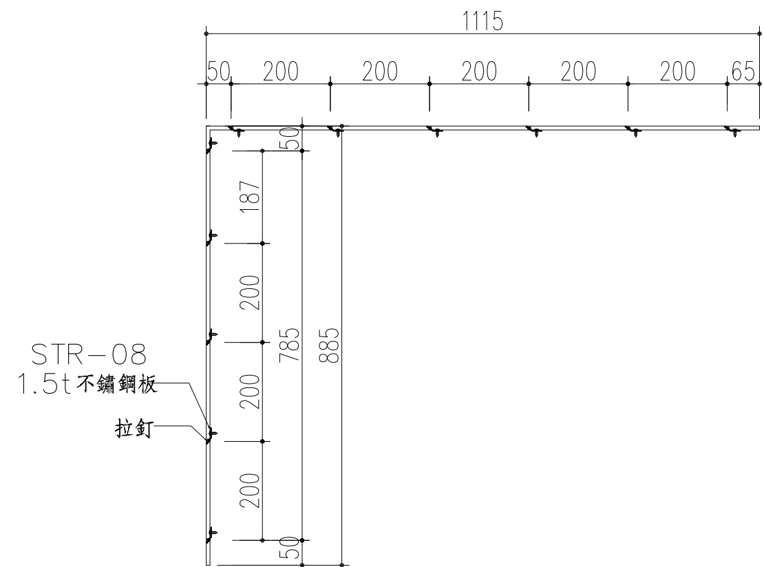
A剖圖
