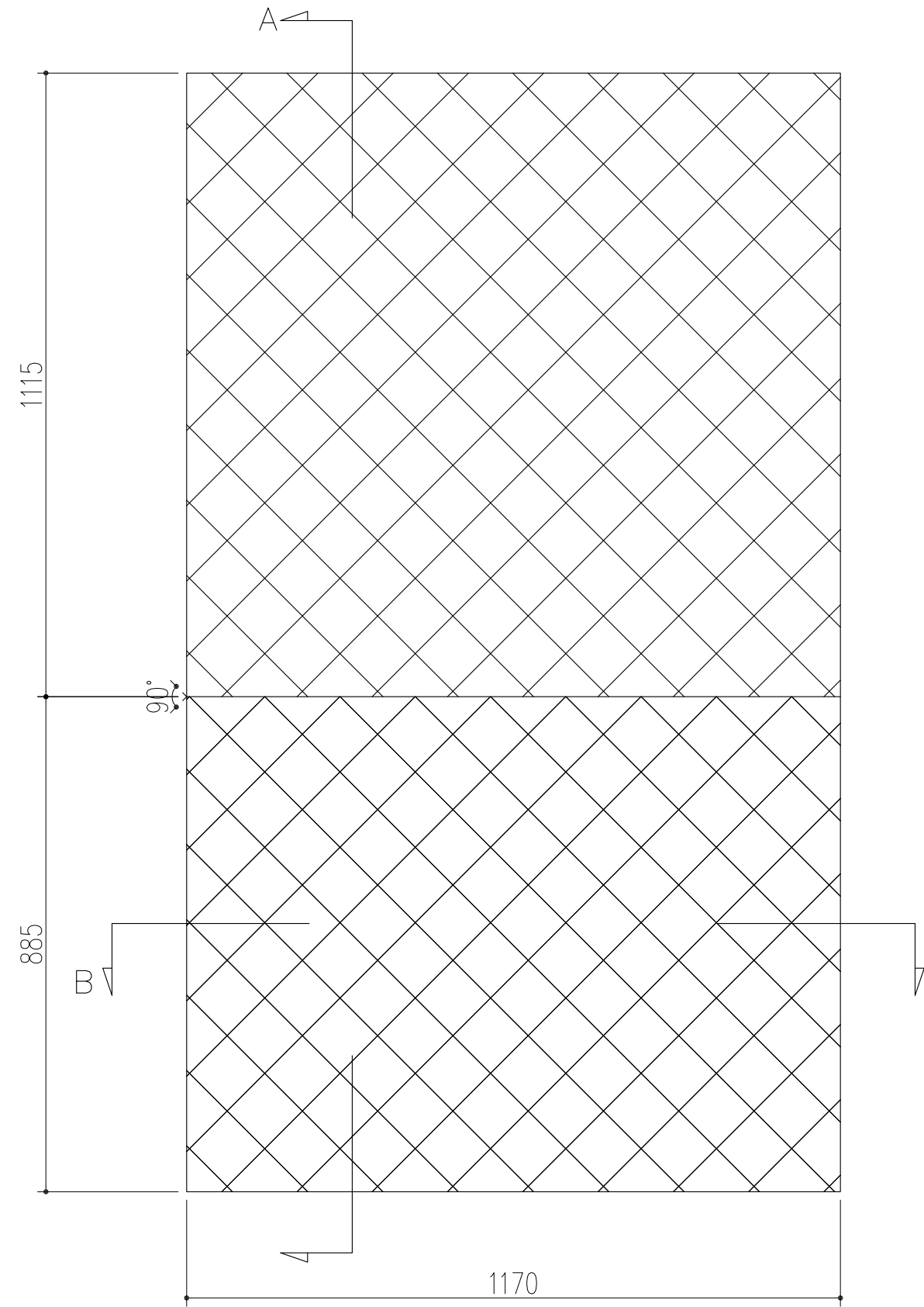
鋁擴張網立面圖
