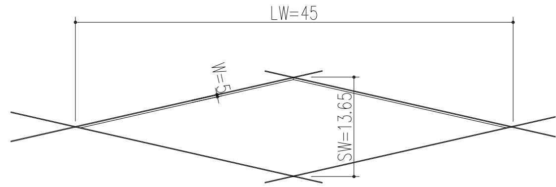
鋁擴張網平面圖
