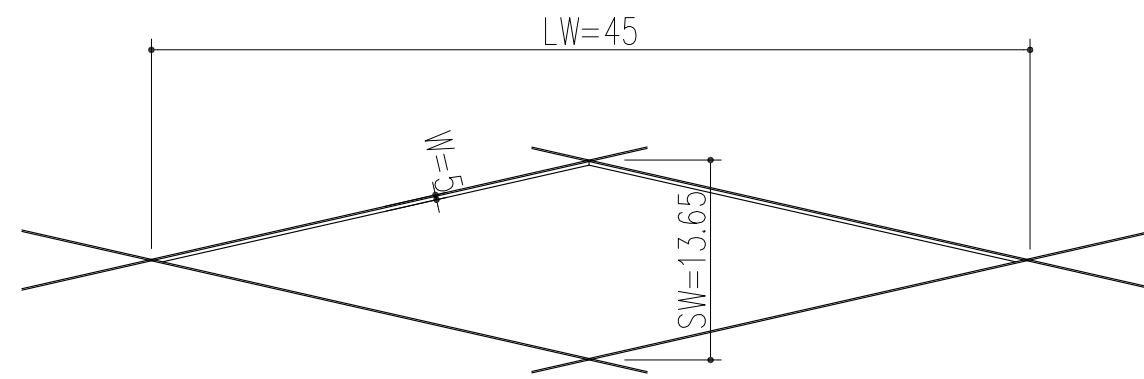
鋁擴張網平面圖
