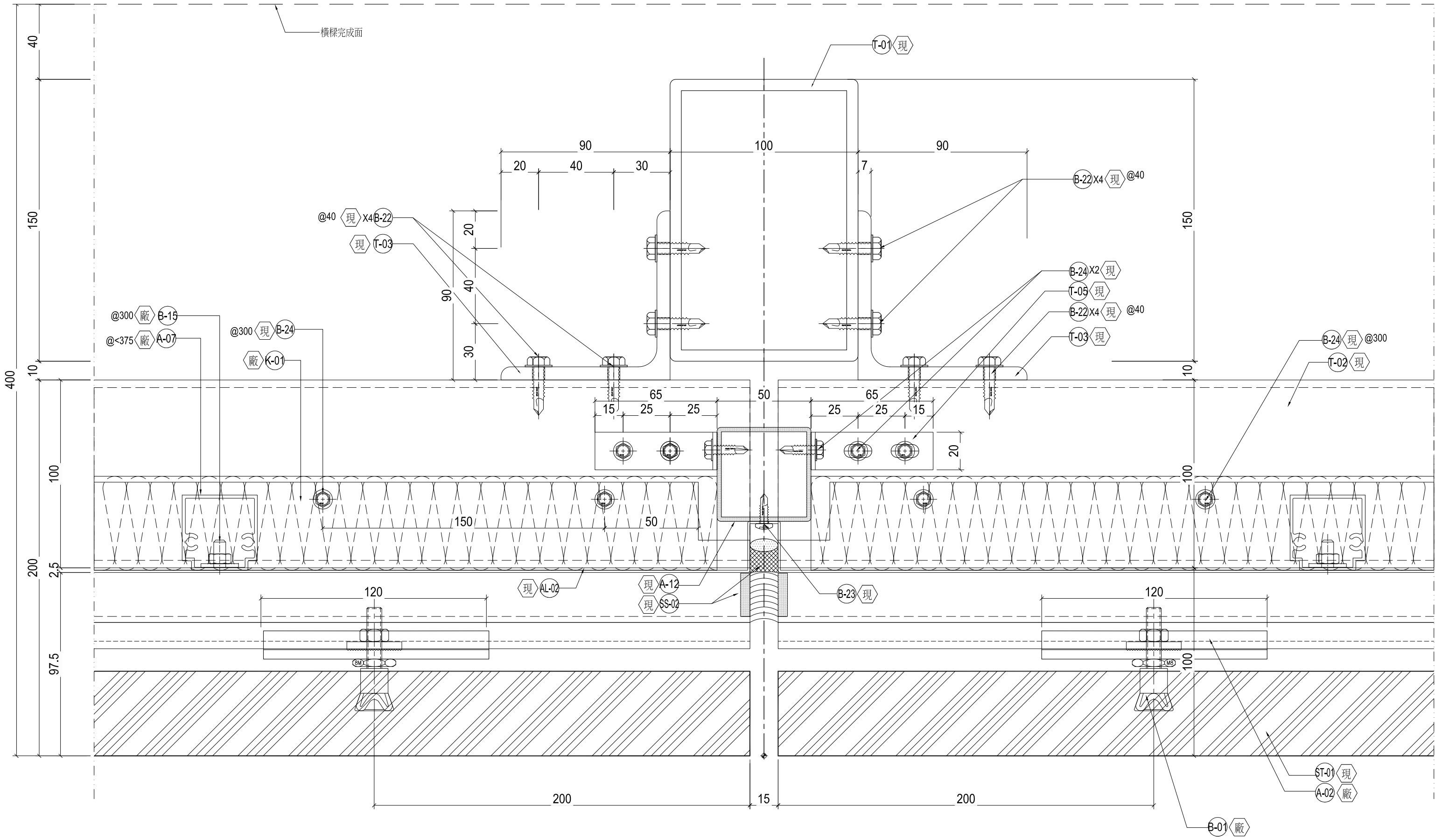
1 石材施工大樣詳圖 SCALE: (A3)
